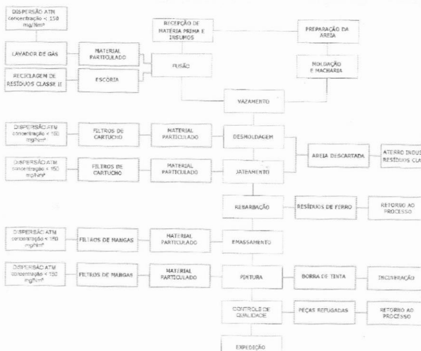
Fig. 2 – Fluxograma com ilustração do processo produtivo.
