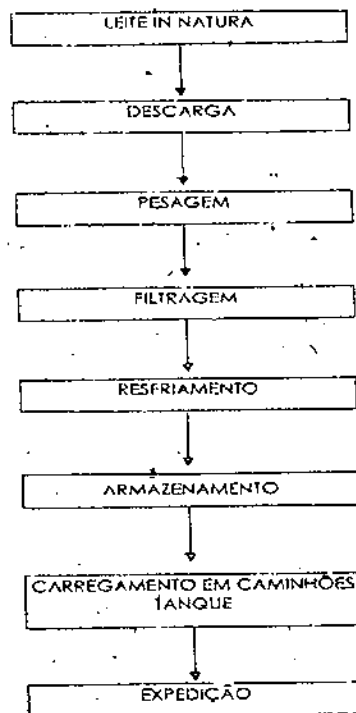
Figura 2- Fluxograma do processo produtivo
