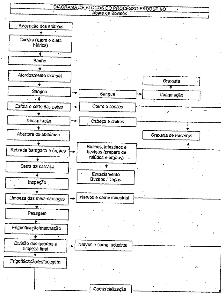
Figura 2: Fluxograma de abate dos bovinos. Fonte: RADA
