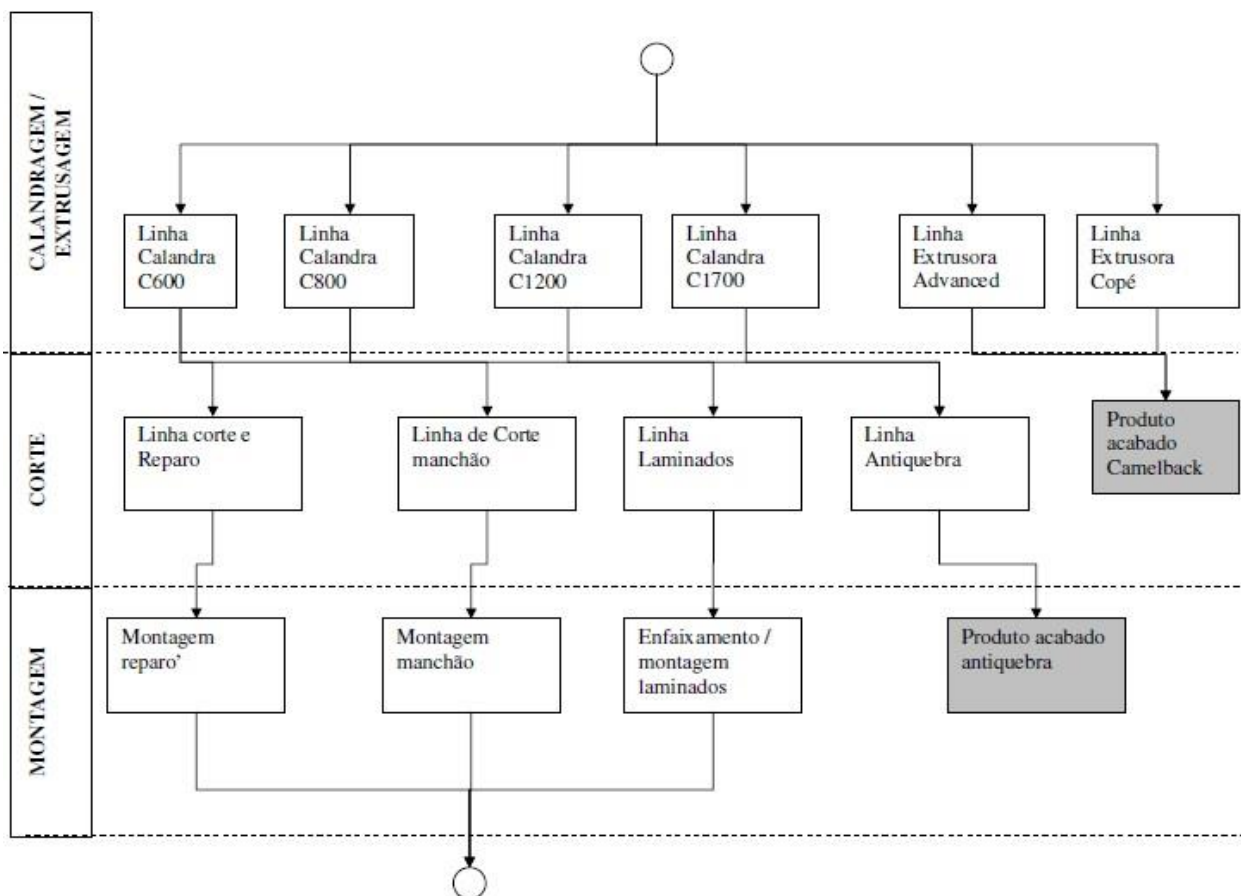
FIGURA 3: Fluxograma do processo produtivo 2.
