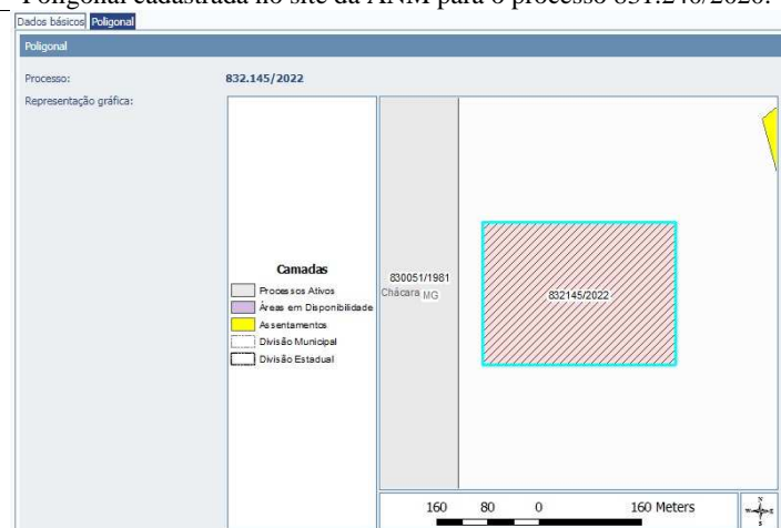
Poligonal cadastrada no site da ANM para o processo 832.145/2022.
