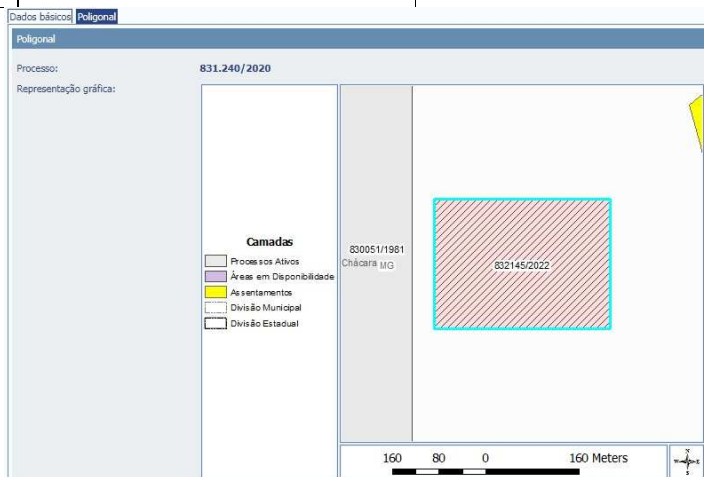
Poligonal cadastrada no site da ANM para o processo 831.240/2020.
