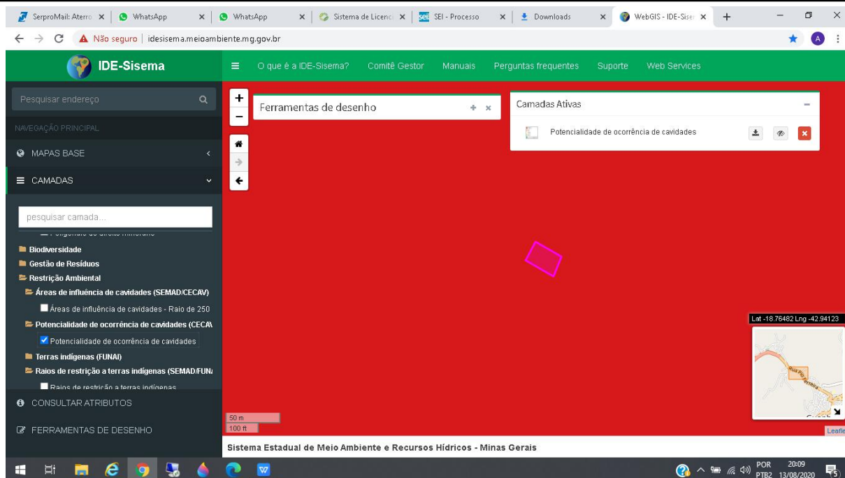
Figura 02: Imagem da área da propriedade constando o muito alto potencial de ocorrência de cavidades.
