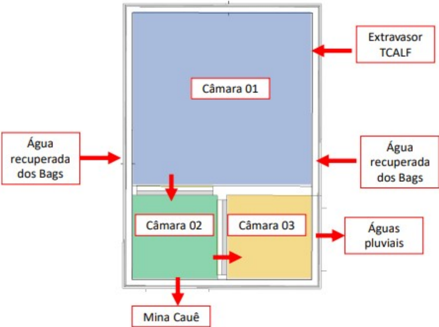
FIGURA 02. Reservatório de água de reuso Fonte: Memorial descritivo da ETA – IC 09.
