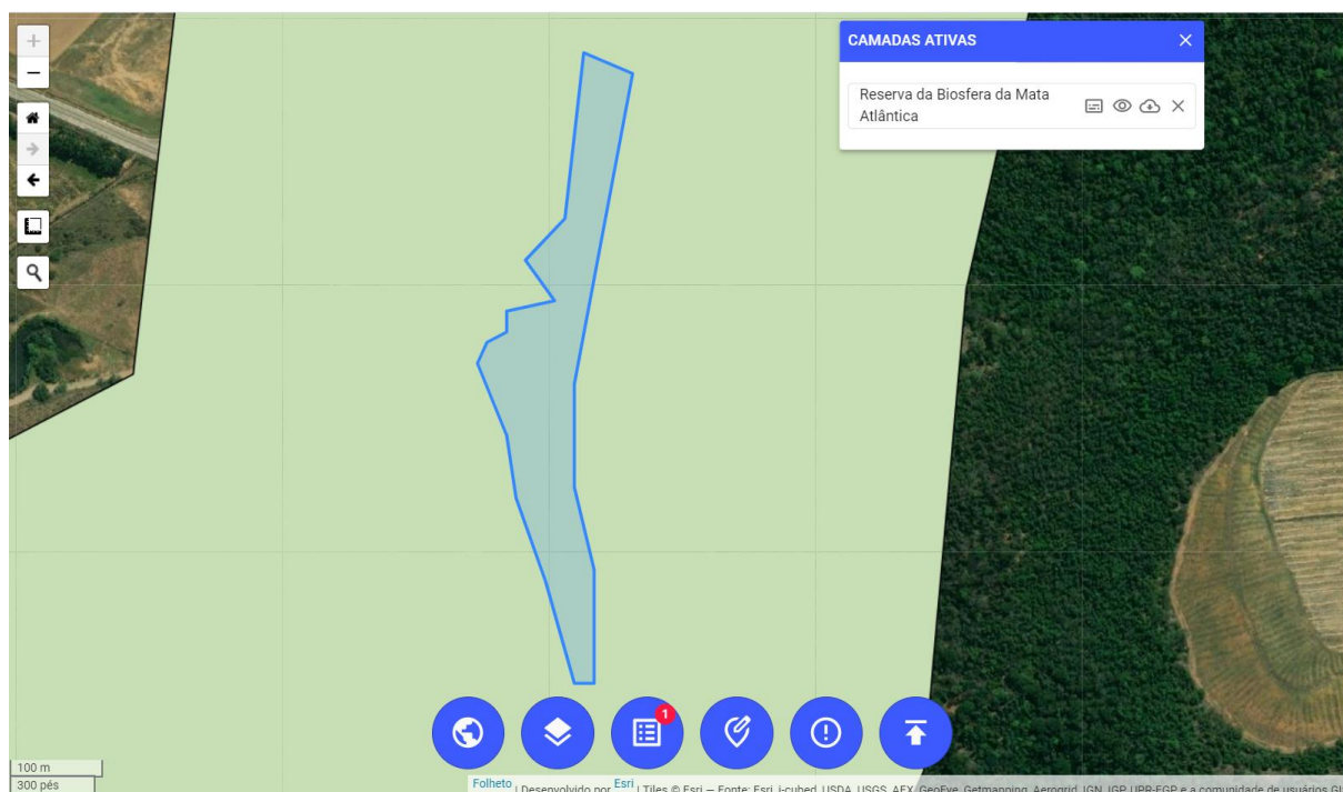
Figura 02: Poligonal da ADA do empreendimento localizada na Reserva da Biosfera da Mata Atlântica. Fonte: IDE-SISEMA (acessado em 19/09/2022).
