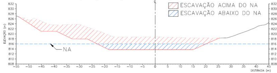
Figura 6: Etapas 3 e 4 do sequenciamento construtivo do sump. Fonte: Walm, 2023.
