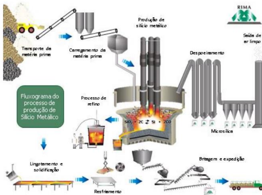
Figura 02: Fluxograma de Produção
