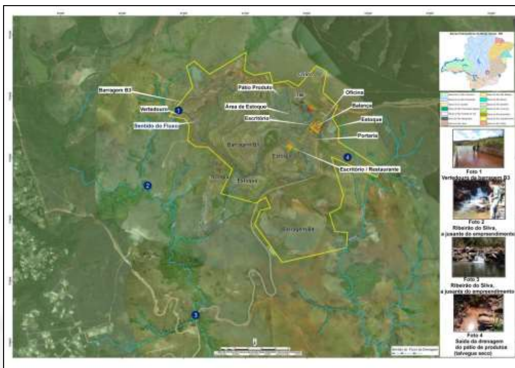
Figura 18 Imagem satélite do empreendimento destacando o alvo do licenciamento, contorno amarelo (retomada de finos com lavra de room, beneficiamento e disposição de rejeito em pilha), na Mina Tanque Seco e os pontos de monitoramento hídrico (azul escuro).
