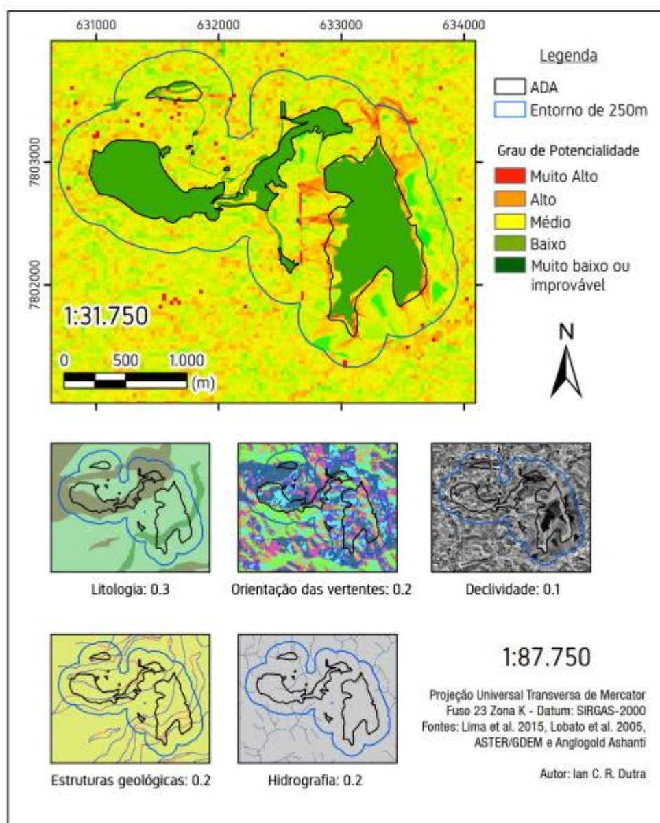
Figura 23: Mapa do potencial espeleológico baseado na Análise de Decisão Multicritérios (ADM). Fonte: Relatório de Prospecção Espeleológica: Mina Cuiabá. GEOIT Consultoria Ambiental, 2018.
