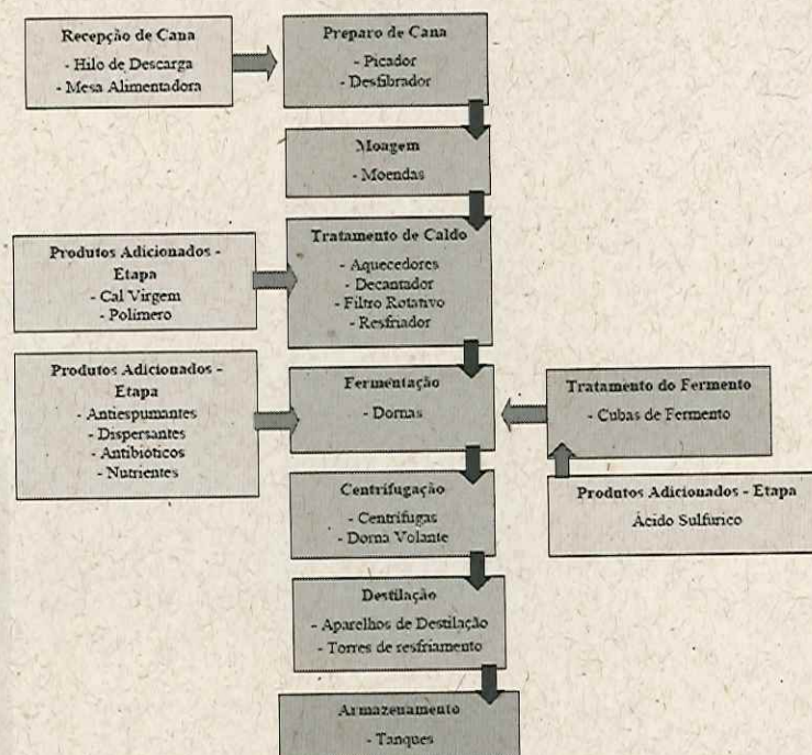
Imagem 01: Fluxograma do processo produtivo.
