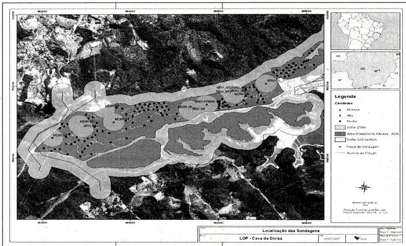
Figura 10: Mapa de Localização das praças de sondagem e dos acessos em relação às cavidades naturais subterrâneas e o perímetro protetivo de 250m (IC protocolo nº 1052707/2017).
