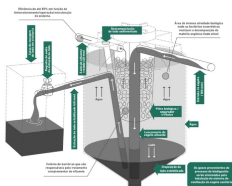
Figura 33 - Sistema Biodigestor Acqualimp
