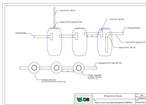
Figura 32 Fossa biodigestor modelo Embrapa Adaptada.
