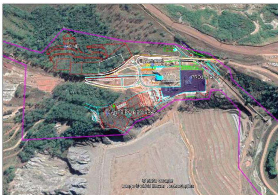
Figura 12- Área prevista para implantação da “Filtragem”. Fonte: EIA
