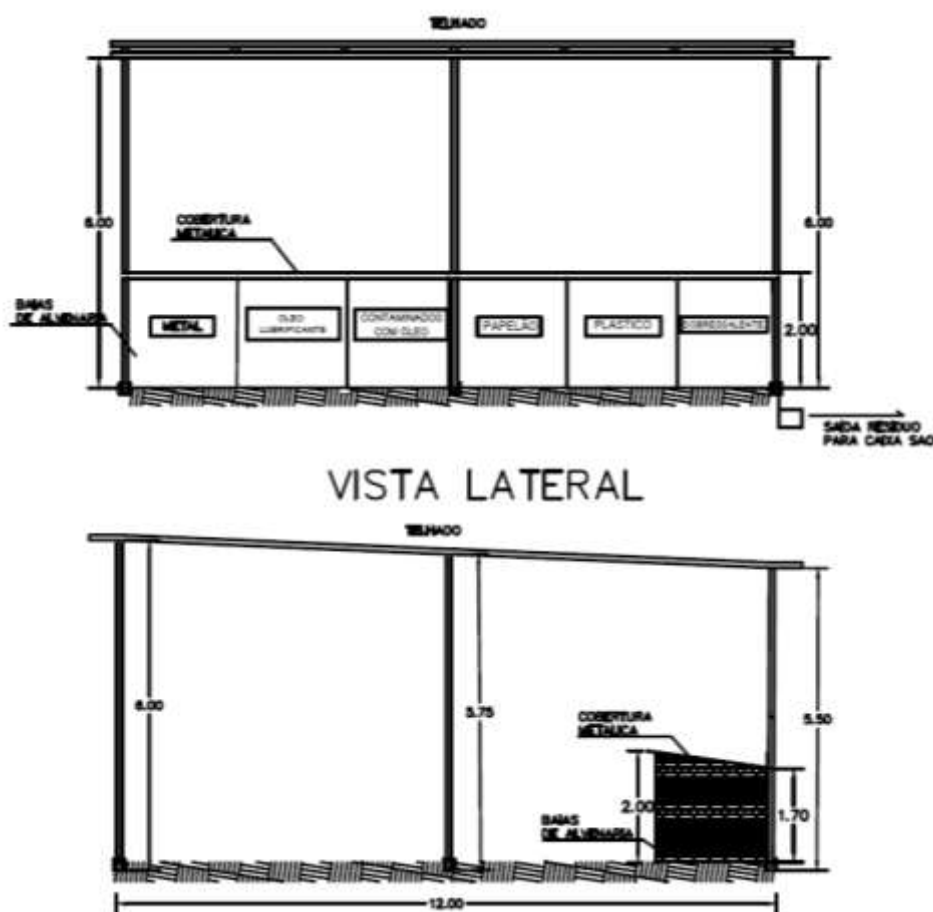
Figura 20: Detalhe do galpão de armazenamento temporário de resíduos sólidos. Fonte: Plano de Gerenciamento de Resíduos Sólidos, 2021.
