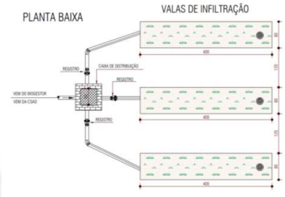
Figura 17: Valas de infiltração para disposição dos efluentes da ETE e CSAO Fonte: Projeto de Disposição Final de Efluentes Tratados, 2021.
