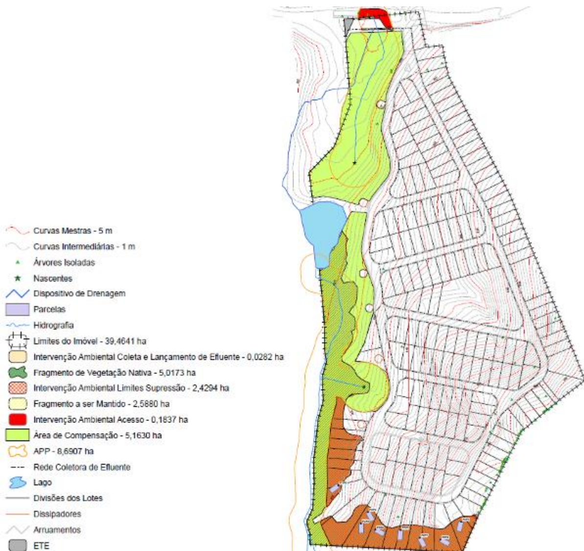
Figura 6 - Intervenções previstas
