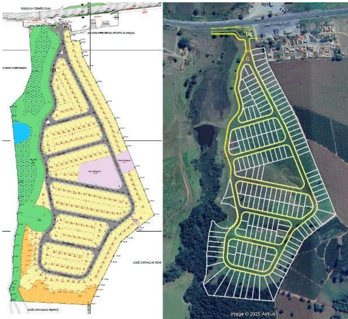
Figura 1 – Arranjo geral do empreendimento
