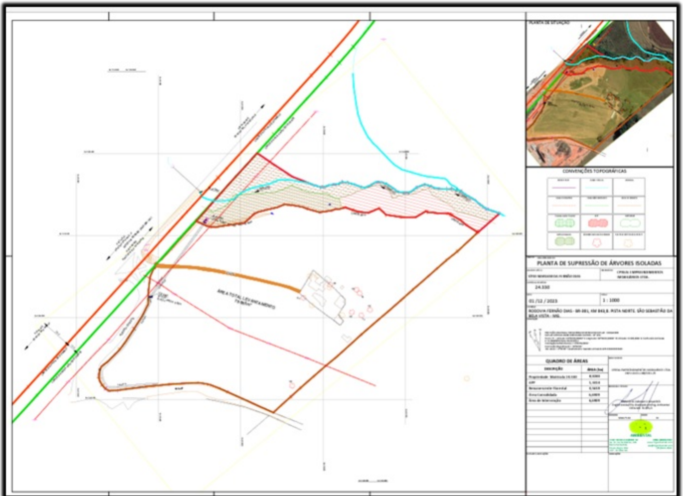
FIGURA 01: Levantamento planimétrico e localização das espécimes requeridas.
